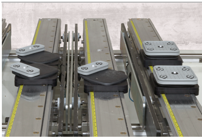
Adapter-Plate AP-S4 con ventosas de bloque VCBL-B para fijar piezas de madera con diferentes geometrías
